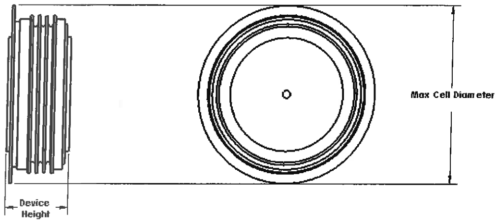
Fig. 2 - Device Nomenclature
